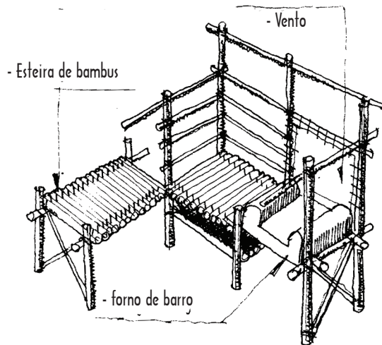
Esteiras e forno de cozinha 2
