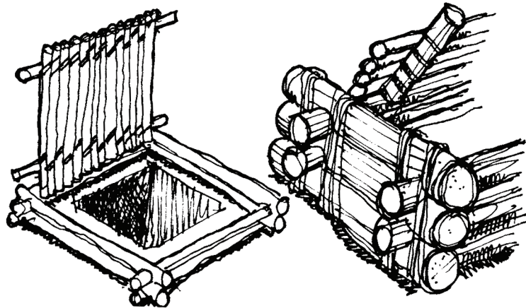
Tampa-fossa de orgânicos
